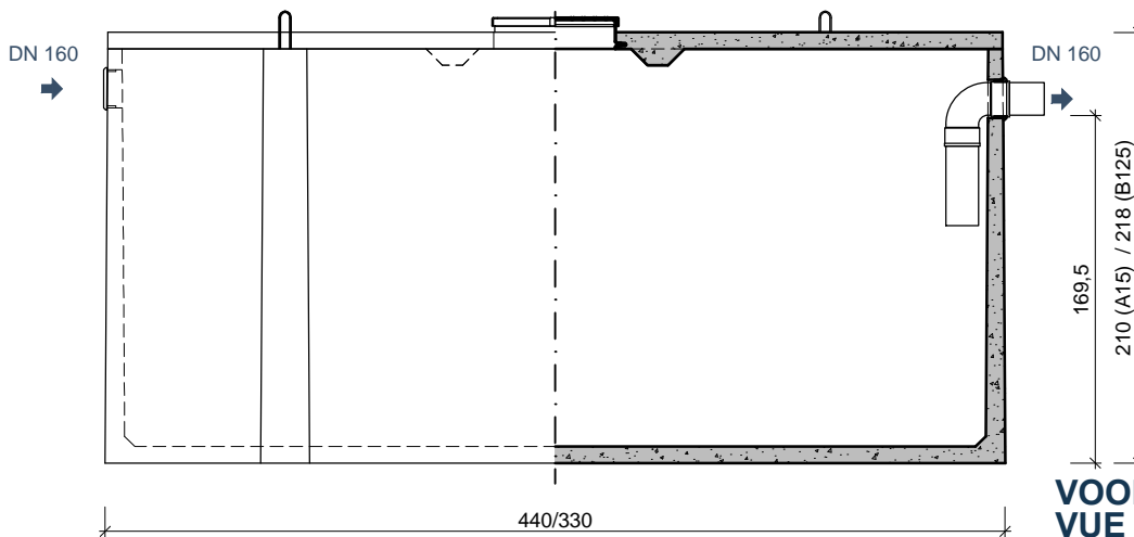
BOVENAANZICHT VUE DE DESSUS
