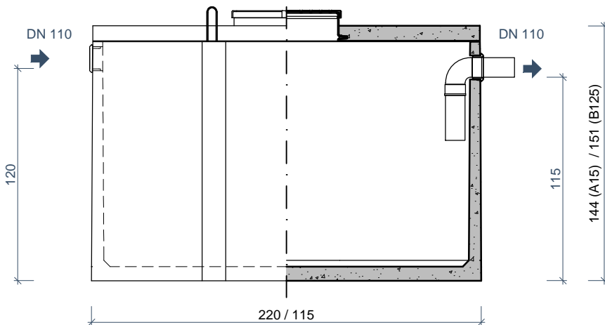
VOORAANZICHT / DOORSNEDE VUE FRONTALE / COUPE
