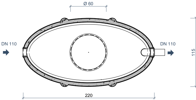
BOVENAANZICHT VUE DE DESSUS
