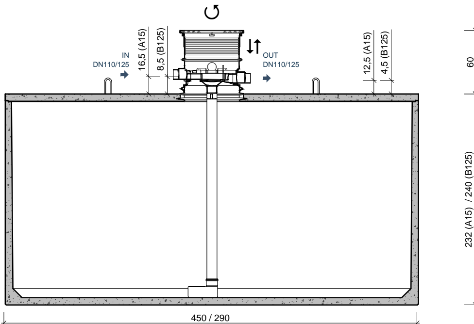
DOORSNEDE COUPE
