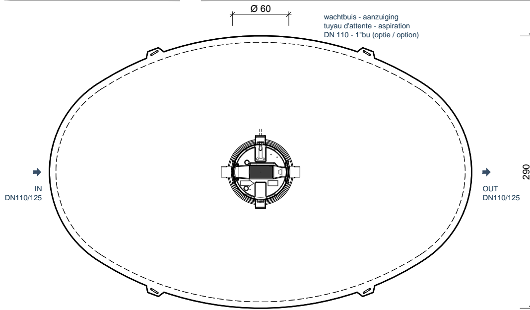
BOVENAANZICHT VUE DE DESSUS
