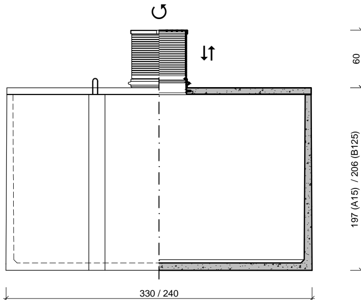
VOORAANZICHT / DOORSNEDE VUE FRONTALE / COUPE
