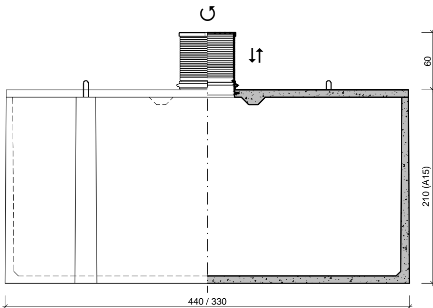
VOORAANZICHT / DOORSNEDE VUE FRONTALE / COUPE
