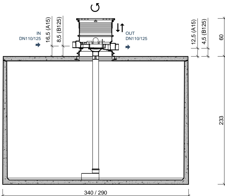
DOORSNEDE COUPE
