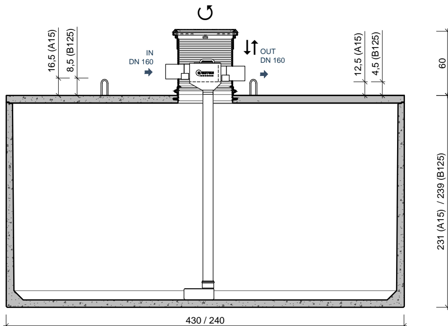
DOORSNEDE COUPE
