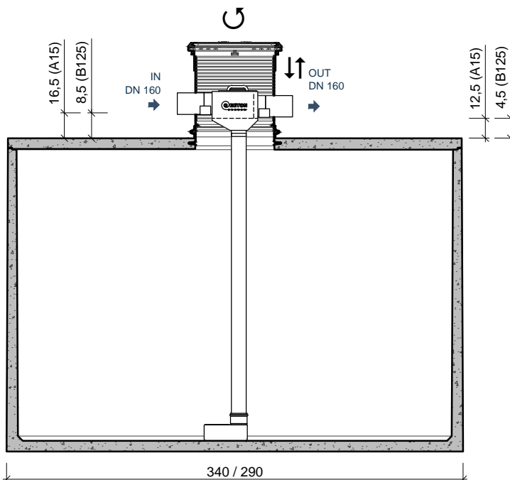
DOORSNEDE COUPE
