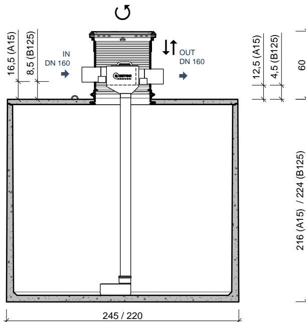
DOORSNEDE COUPE
